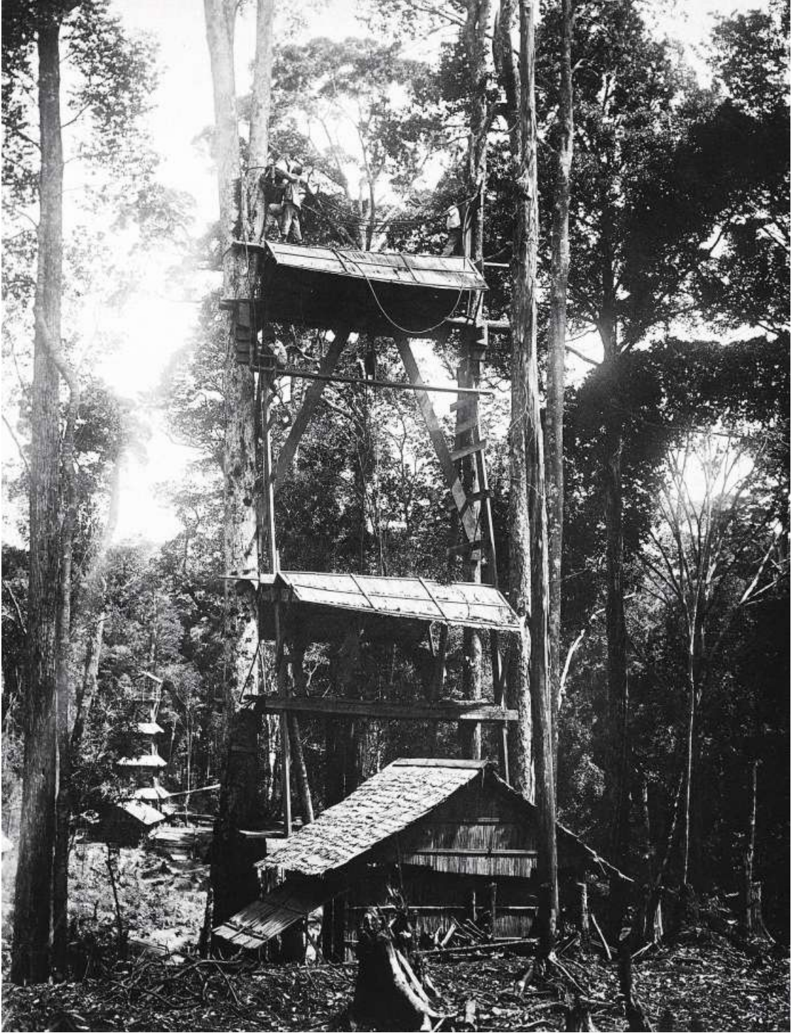
Erdölsuche mit Schweizer Know-how: Bohrung auf Bunyu (heute Indonesien) um 1923. Als Bohrturm dienen zwei Bäume, durch Balken verbunden.
