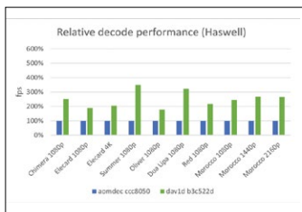
Vergleich der Dekodierleistung unter Haswell- und Zen-Systemen.
