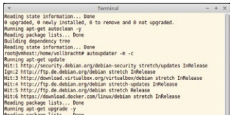
Autoupdater hält Debian-Systeme aktuell.
